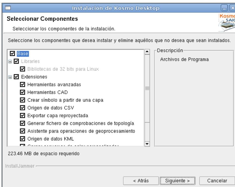
Imagen 19: Linux - Instalador - Instalación personalizada - Seleccionar componentes a instalar
